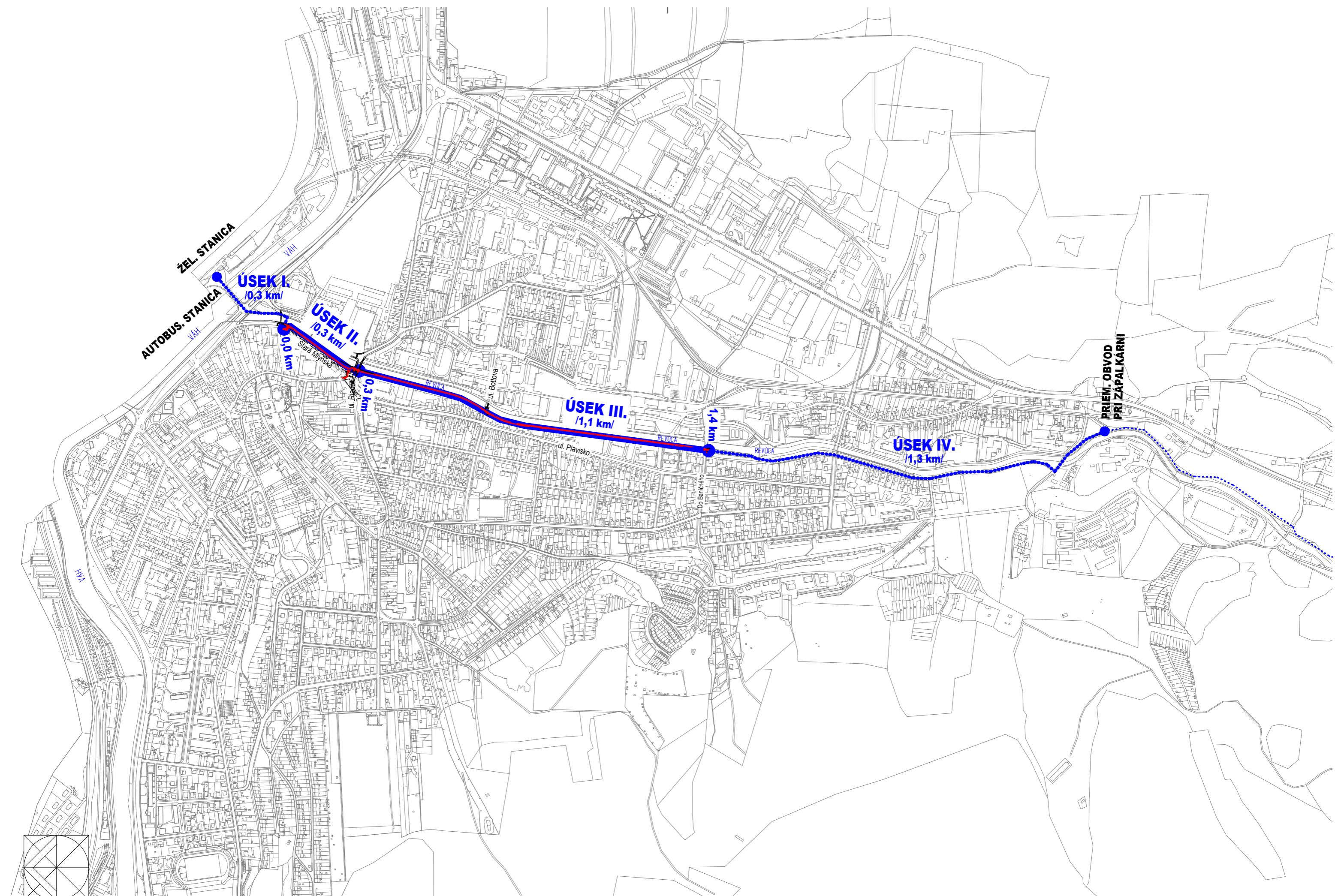
A. SITUÁCIA - NAVRHOVANÁ CYKLISTICKÁ INFRAŠTRUKTÚRA V ÚZEMÍ MESTA RUŽOMBEROK
